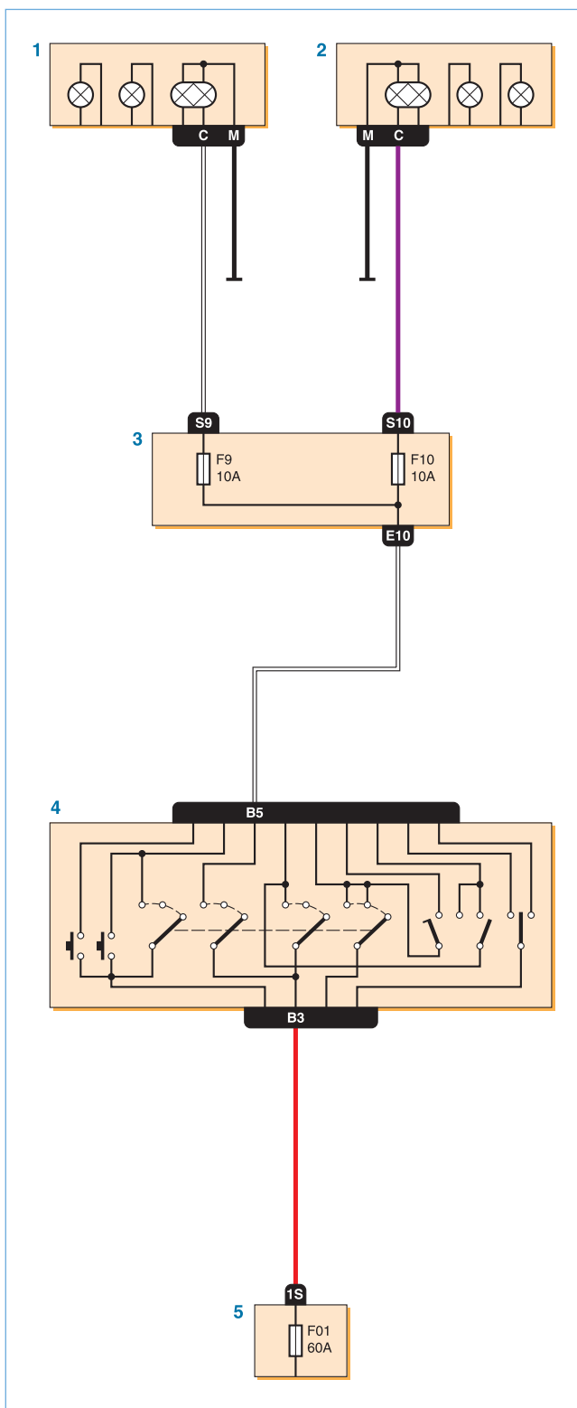
Схема включения ближнего света фар: 1 — левая блок-фара; 2 — правая блок-фара; 3 — монтажный блок предохранителей в салоне; 4 — левый подрулевой переключатель; 5 — монтажный блок реле и предохранителей в моторном отсеке
