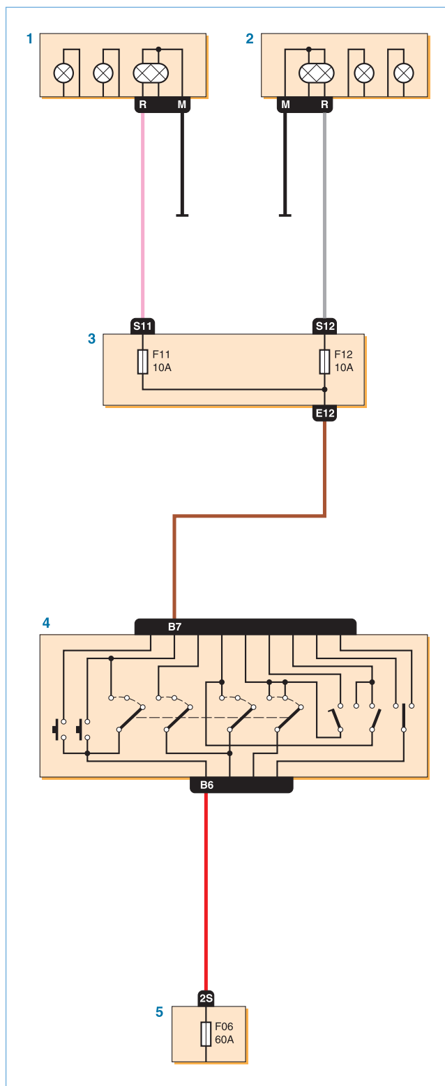
Схема включения дальнего света фар: 1 — левая блок-фара; 2 — правая блок-фара; 3 — монтажный блок предохранителей в салоне; 4 — левый подрулевой переключатель; 5 — монтажный блок реле и предохранителей в моторном отсеке
